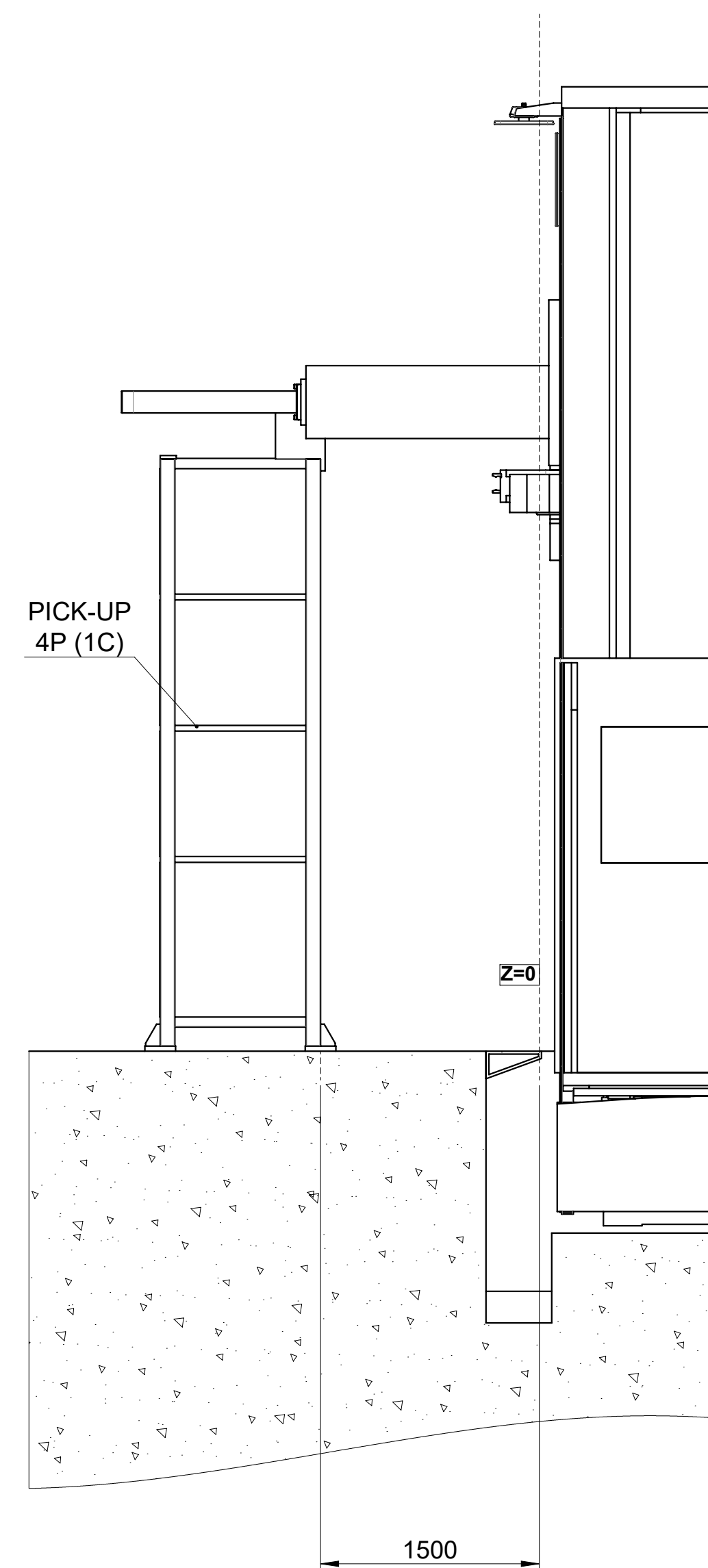
A-A 270°
