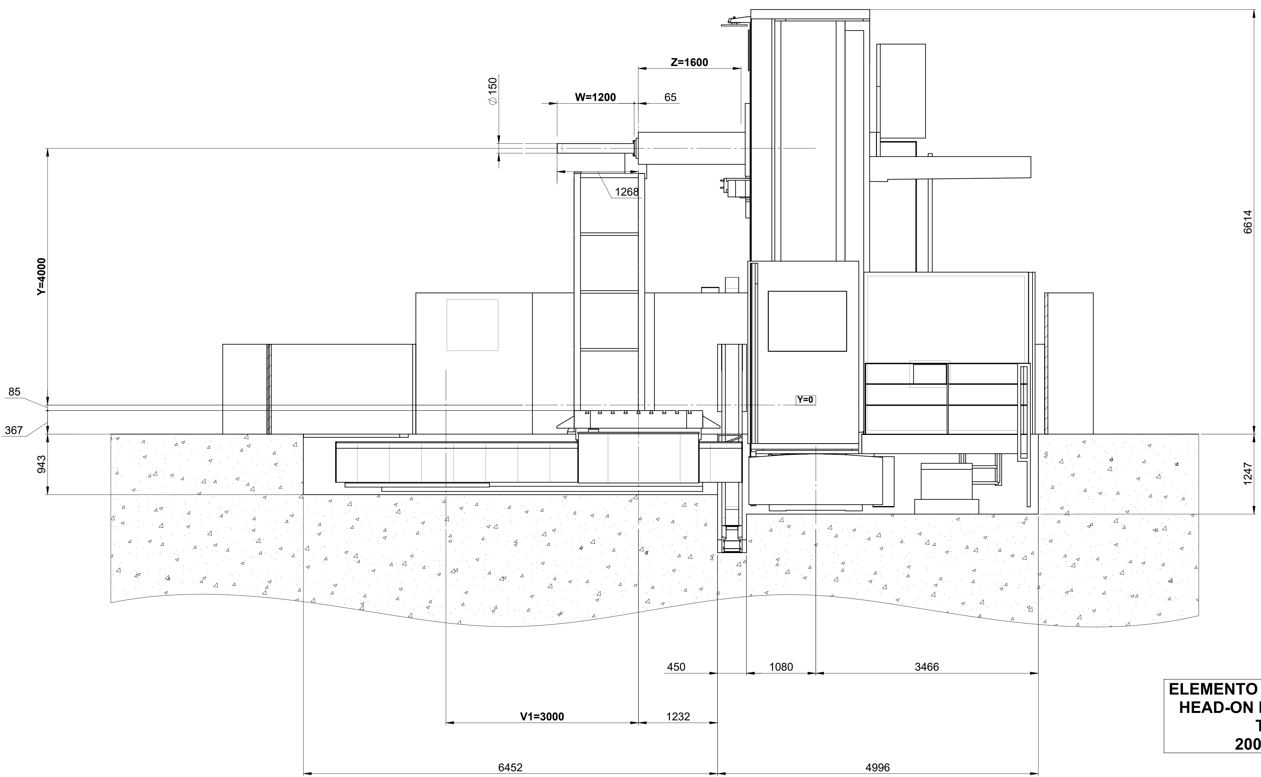
B-B 270°
