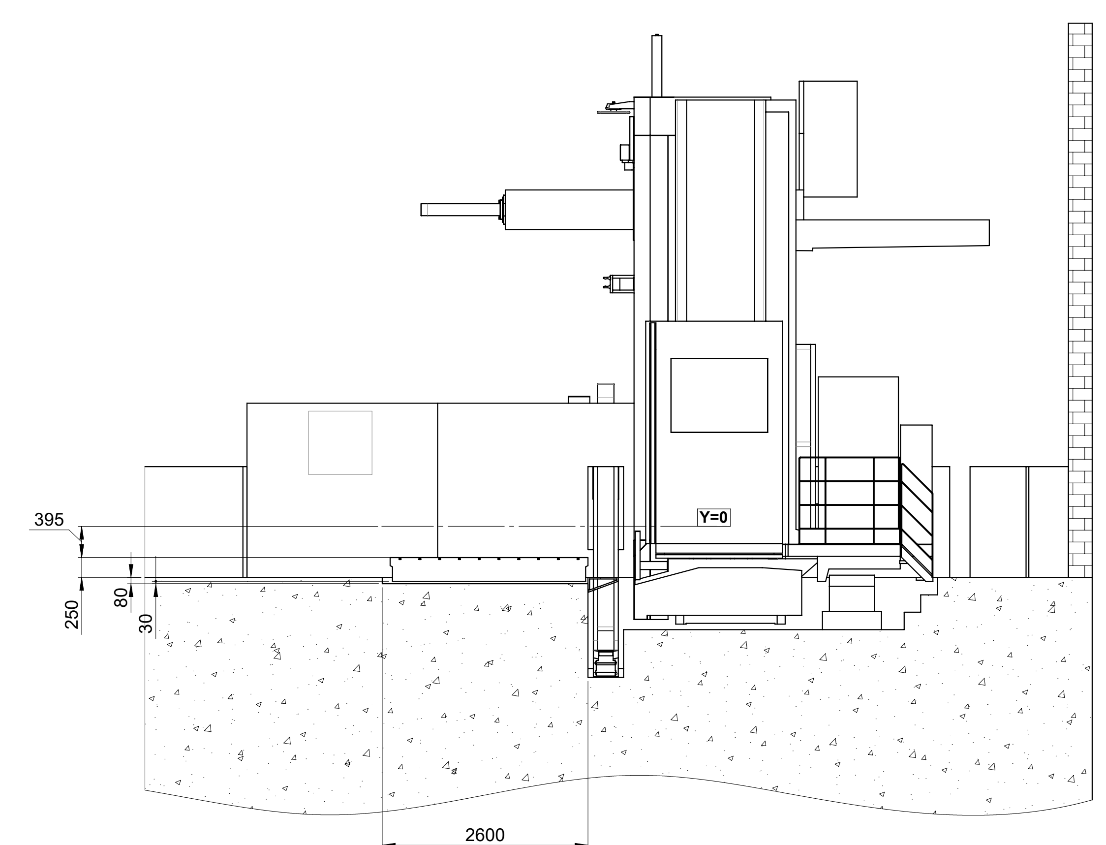
ELEMENTO FRONTALE N°3/ HEAD-ON ELEMENT N°3 PIANO FISSO / FLOOR PLATE 3000X2500
