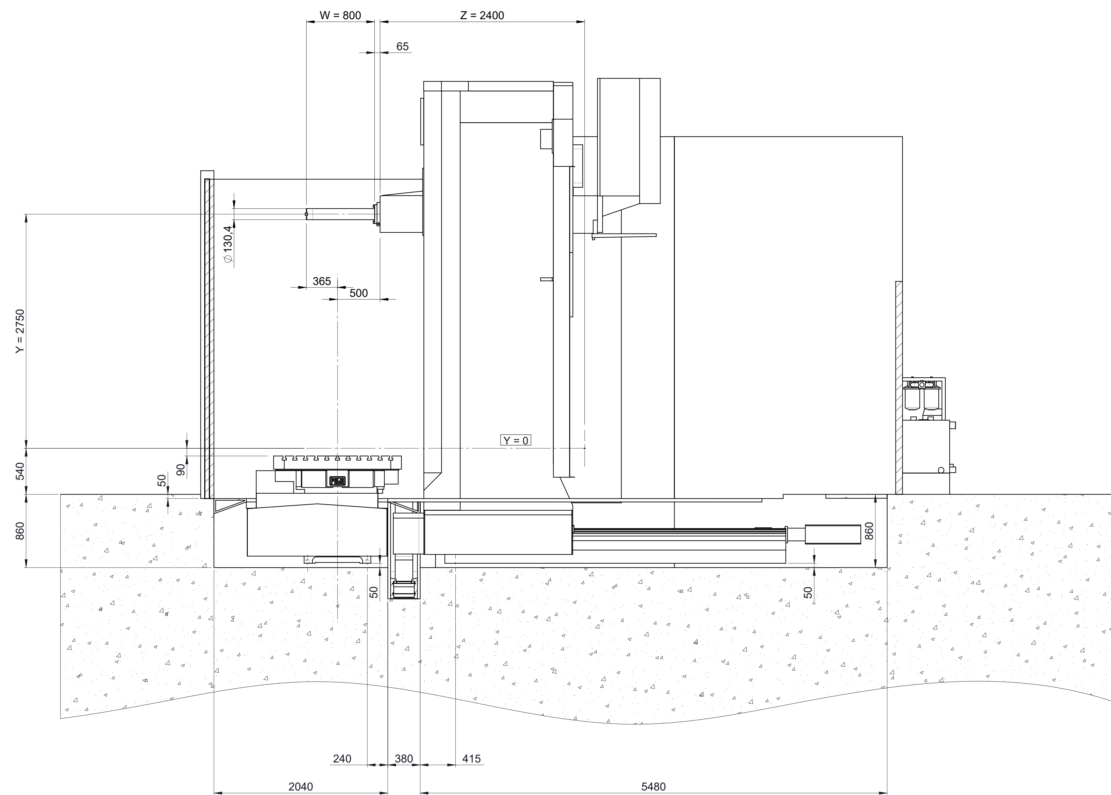
A-A
