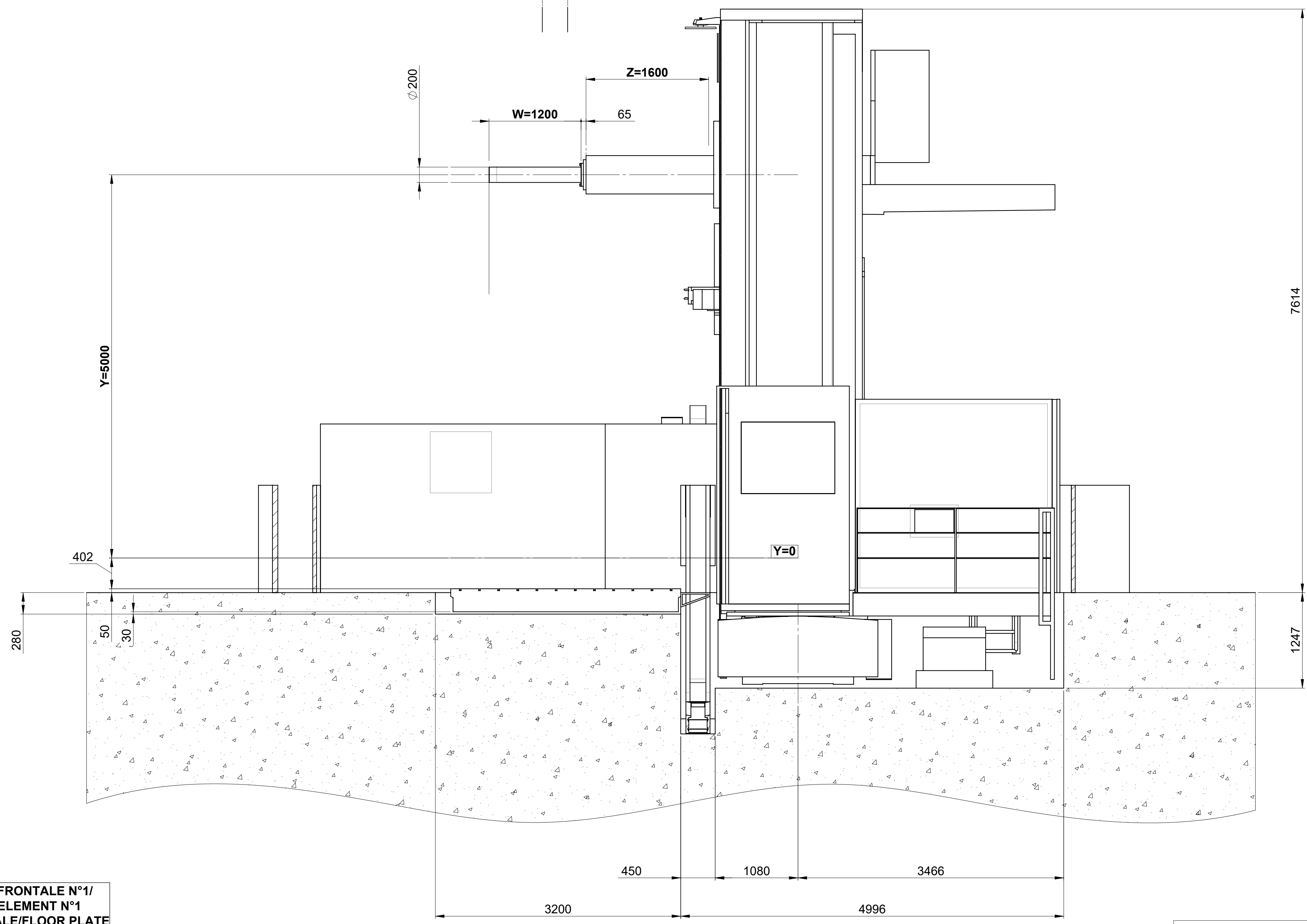
B-B 270°
