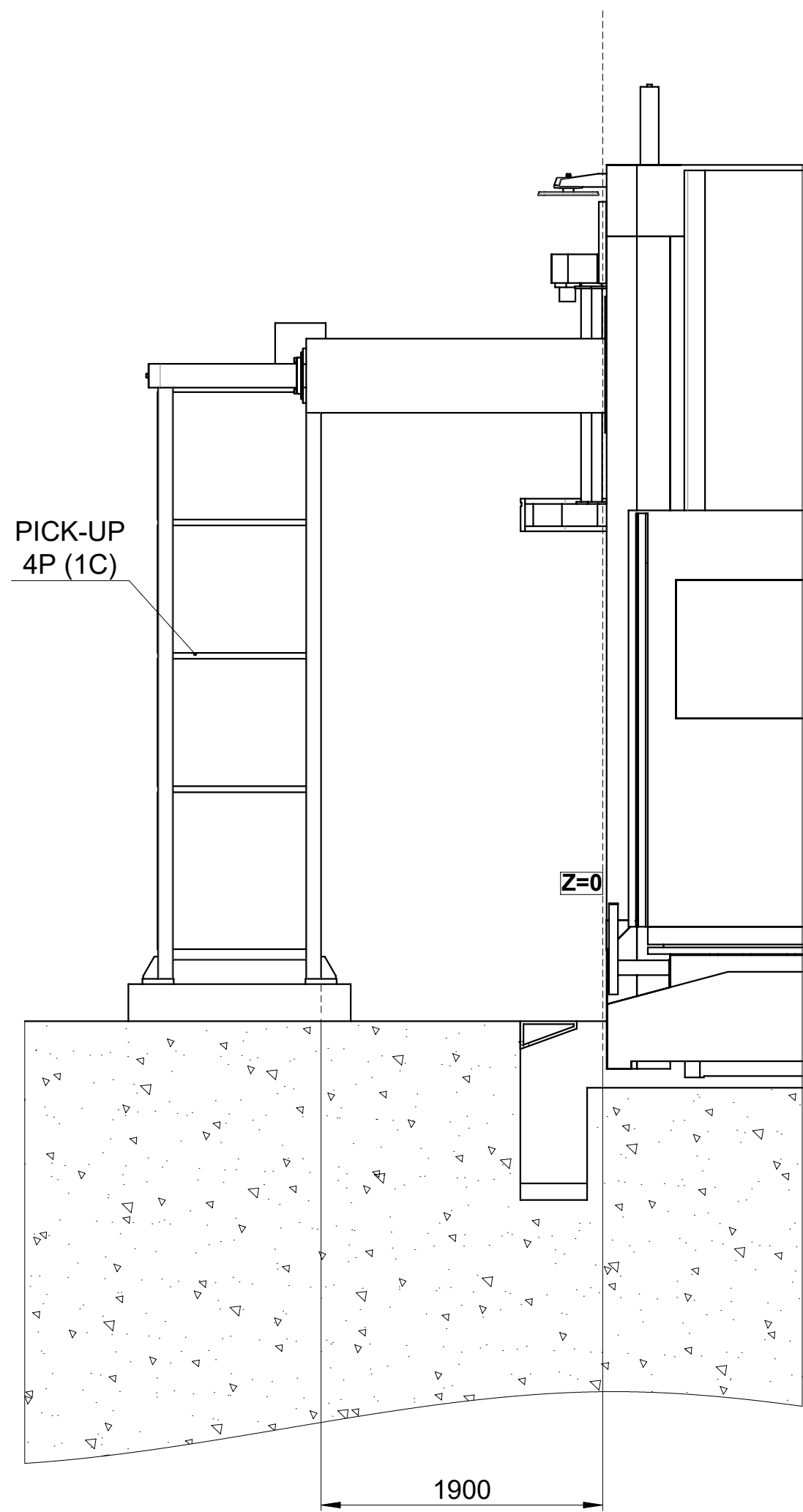
A-A 270°
