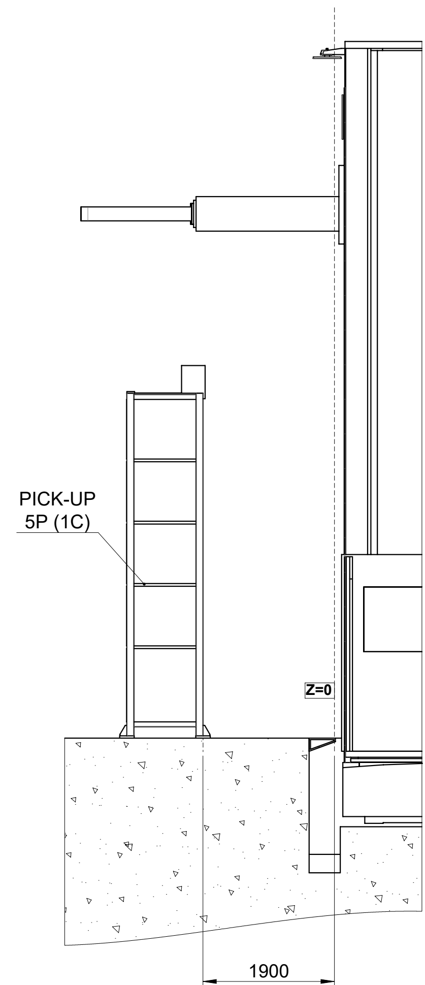
A-A 270°
