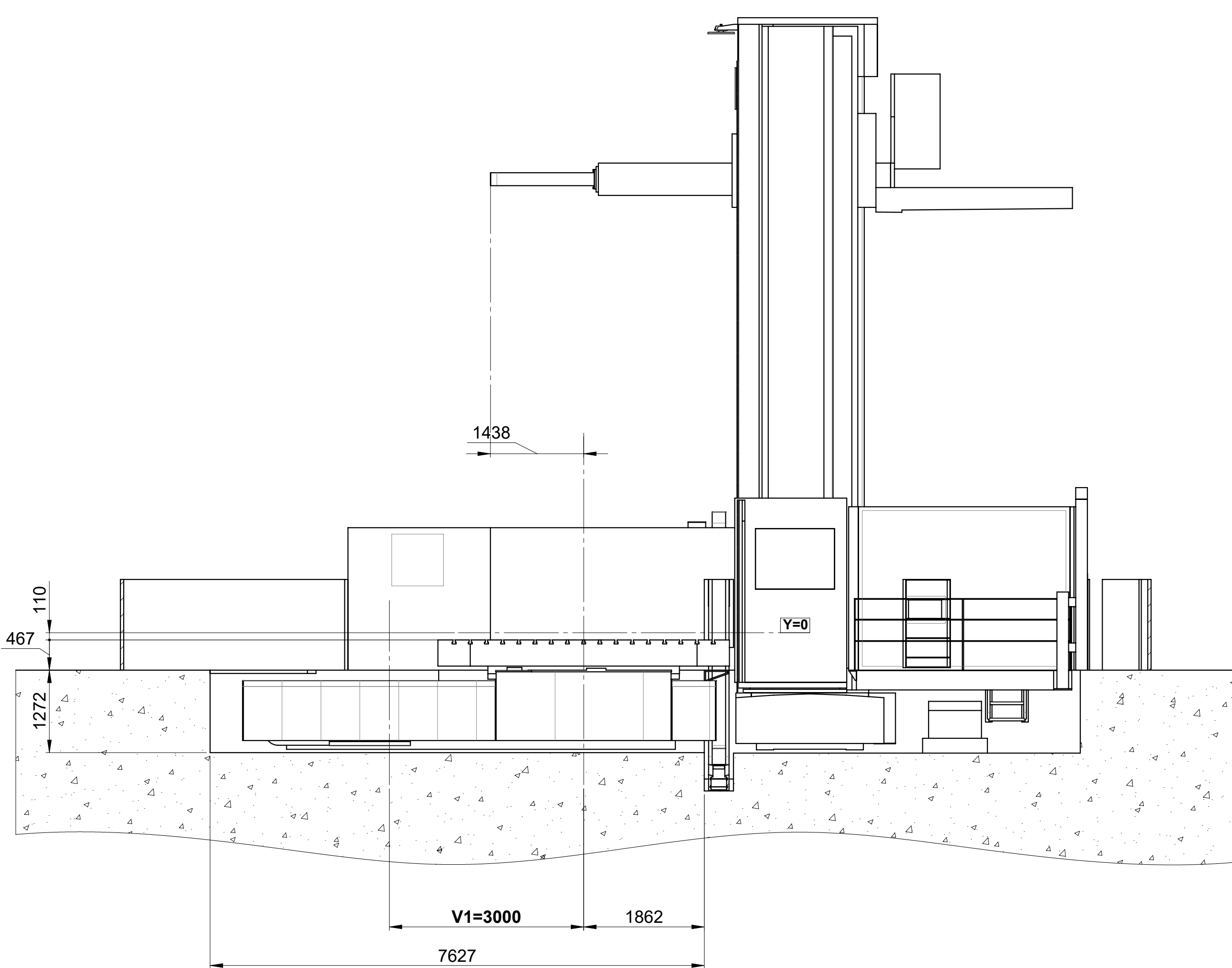
ELEMENTO FRONTALE N°2/ HEAD-ON ELEMENT N°2 TH100 4500x4500
