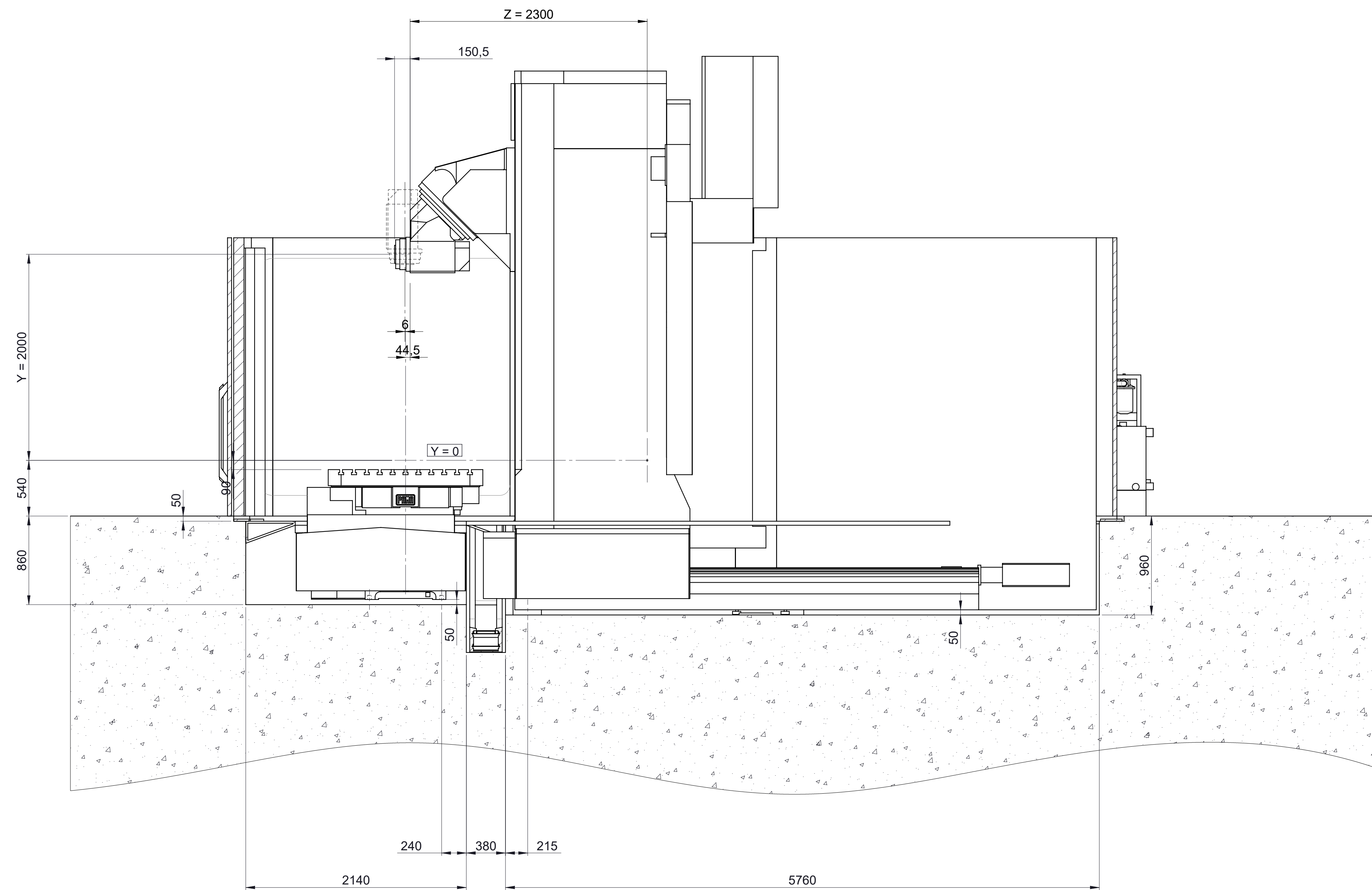
A-A
