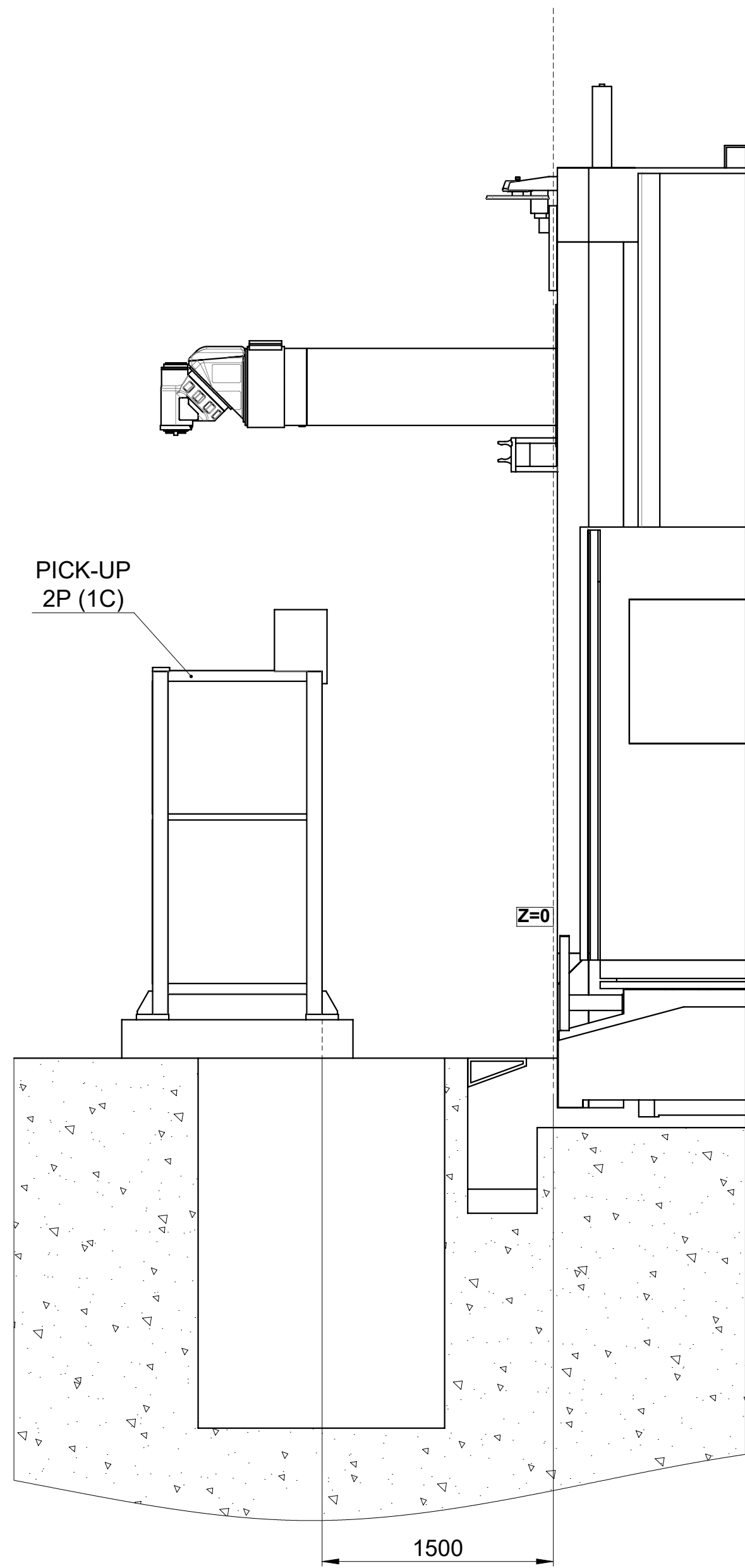
A-A 270°
