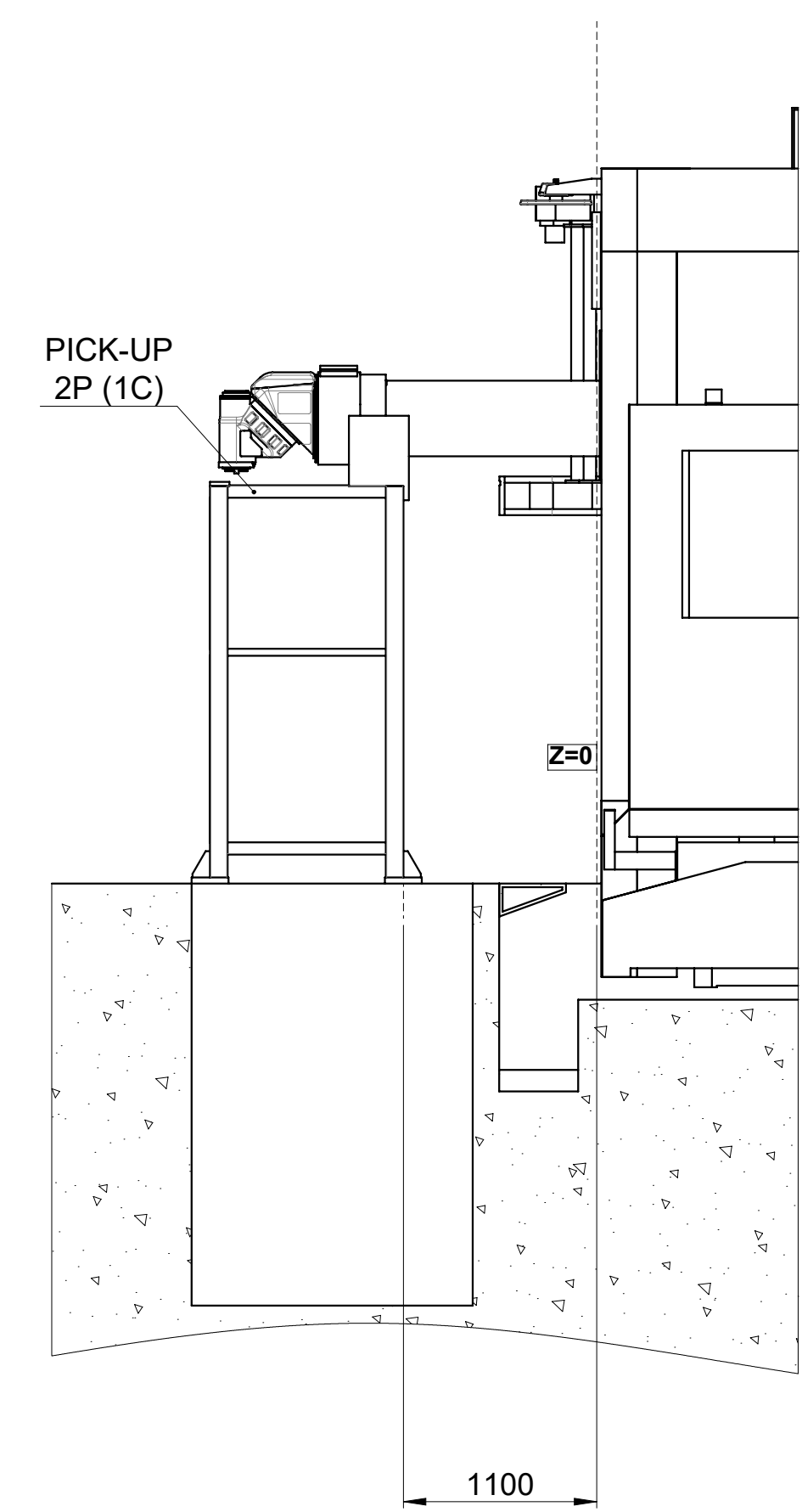
A-A 270°
